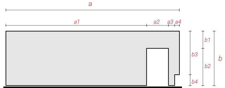
Desfășurare perete dreapta: a : 951cm a1 : 771cm a2 : 120cm a3 : 34cm a4 : 26cm b : 300cm b1 : 95cm b2 : 205cm b3 : 240cm b4 : 60cm
