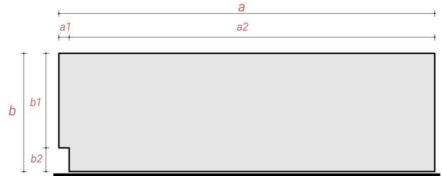
Desfășurare perete stânga: a : 951cm a1 : 26cm a2 : 925cm b : 300cm b1 : 240cm b2 : 60cm
