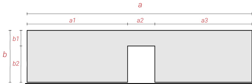
Desfășurare perete intrare: a : 1320cm a1 : 590cm a2 : 160cm a3 : 570cm b : 300cm b1 : 90cm b2 : 210cm
